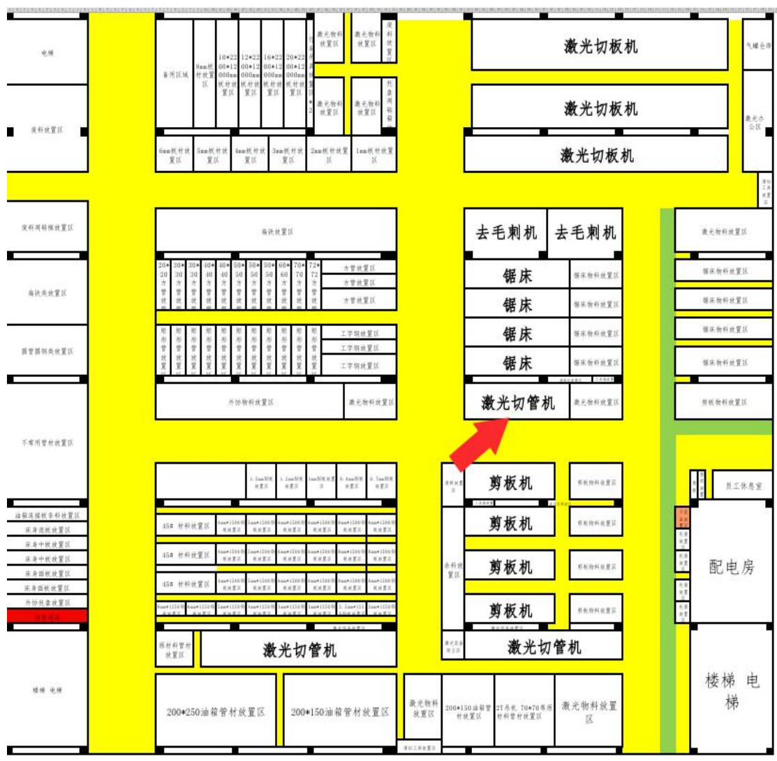
图 1：车间示意图
